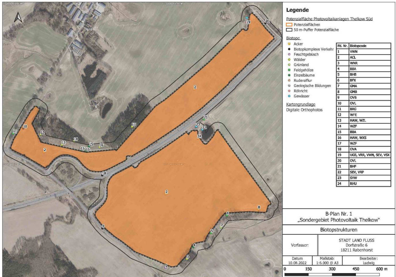
Abb. 24: Biotopstrukturen im Untersuchungsgebiet (HELLWEG & HÖPFNER 2026)
