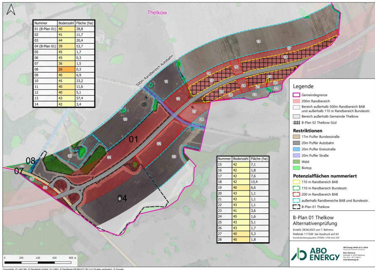
Abb. 1: Bodenwertzahlen im Plangebiet und auf angrenzenden Flächen (ABO ENERGY 2025)
