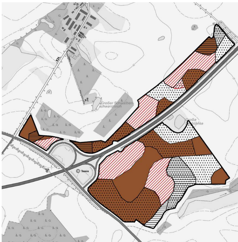
Abb. 25: Bodensystematische Einheiten im Plangebiet (PÄTZOLD 2025)
