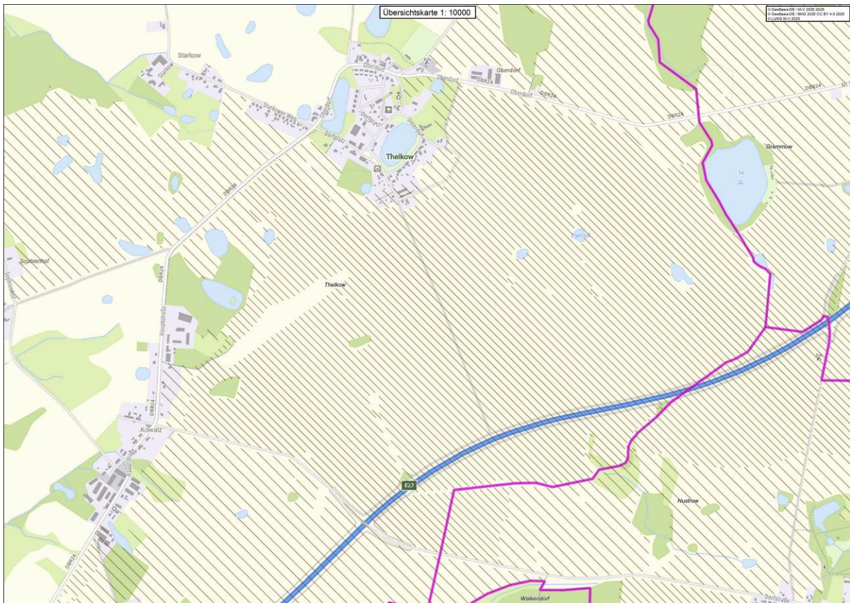
Abb. 4: Rastgebiete für Zugvögel (schraffierte Flächen) (© GeoBasis-DE/ M-V 2025)
